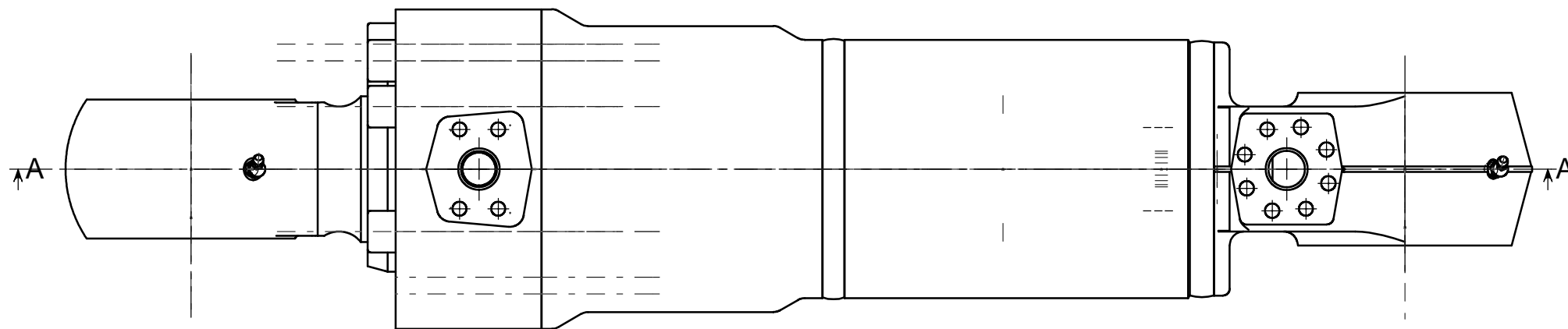
A-A (1 : 3)
